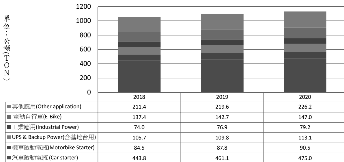
磷酸鐵鋰電池替代鉛酸電池的市場規模
